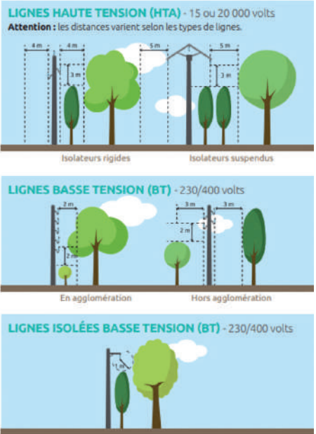
Distances à la construction des lignes électriques (norme NF C 11-201)
